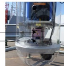
【測定部分】 線量計 CdZnTe半導体検出器
