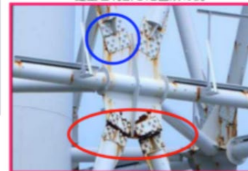
破断及び変形と判断した箇所の例
