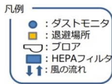
構台、前室、下段フロア平面イメージ
