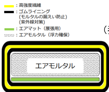
養生バッグ概略構造 (断面)
