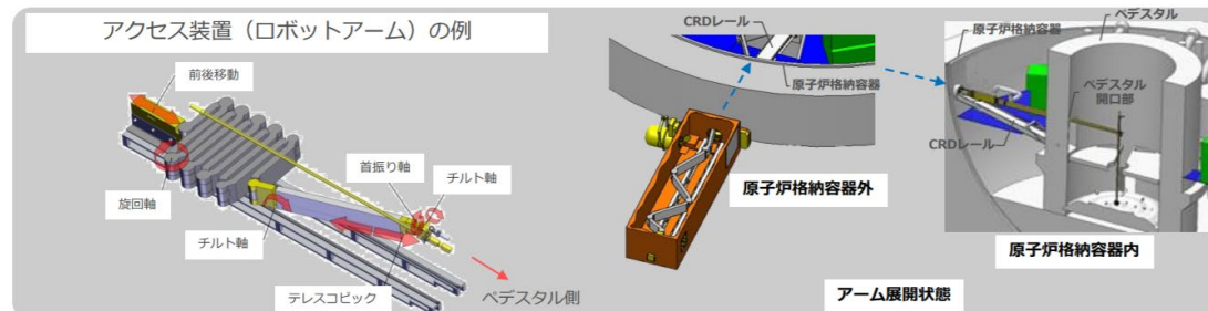
(初期段階の燃料デブリ取り出しのイメージ)
