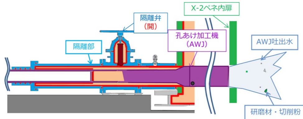
AWJ穿孔作業のイメージ
