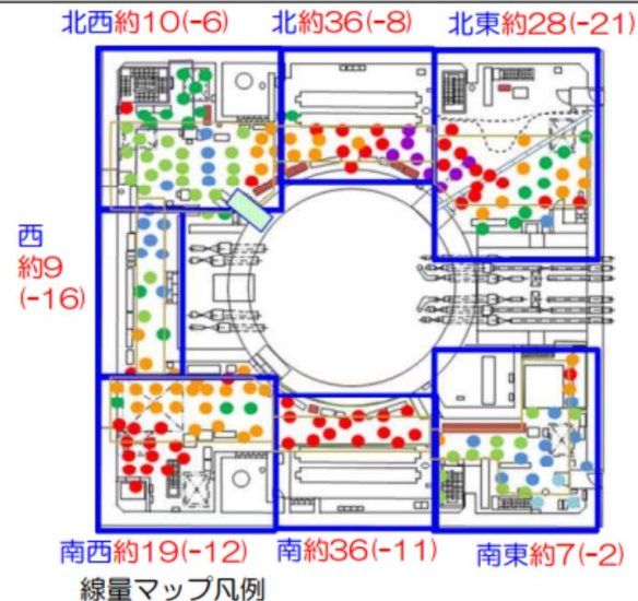
空間線量率 (2015年7月)
