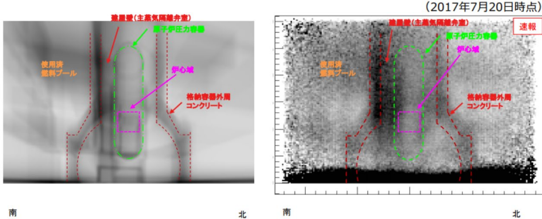
シミュレーションによる物質分布（密度長）の評価 (炉心域、および炉底部に燃料デブリありのケース)
