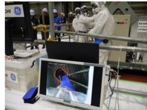
手前モニタを見ながら干渉物を避けホースを降下させる
