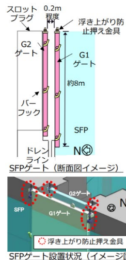
SFPゲート設置状況 (イメージ図)
