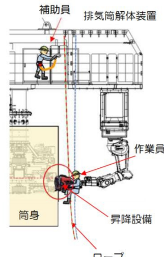
昇筒イメージ
