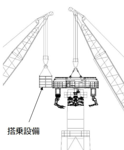
クレーンで吊った搭乗設備を排気筒に近づける
