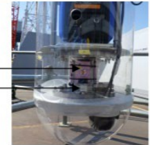
【測定部分】 線量計 CdZnTe半導体検出器
