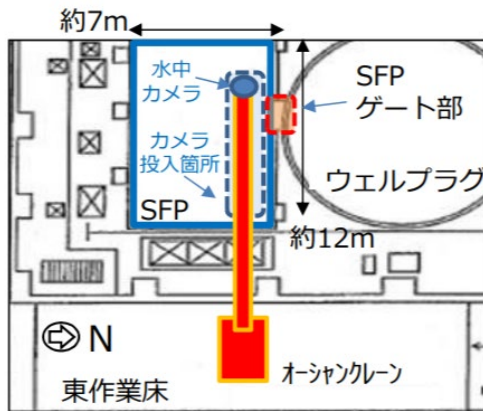
干渉物調査 (平面図) のイメージ
