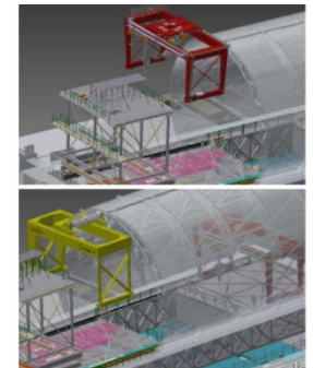
ガータ上吊り込みイメージ
