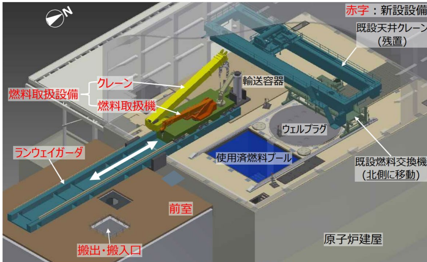
燃料取扱設備概念図 (鳥瞰図)
