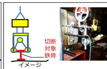
図5 ワイヤソー (今回追加)
