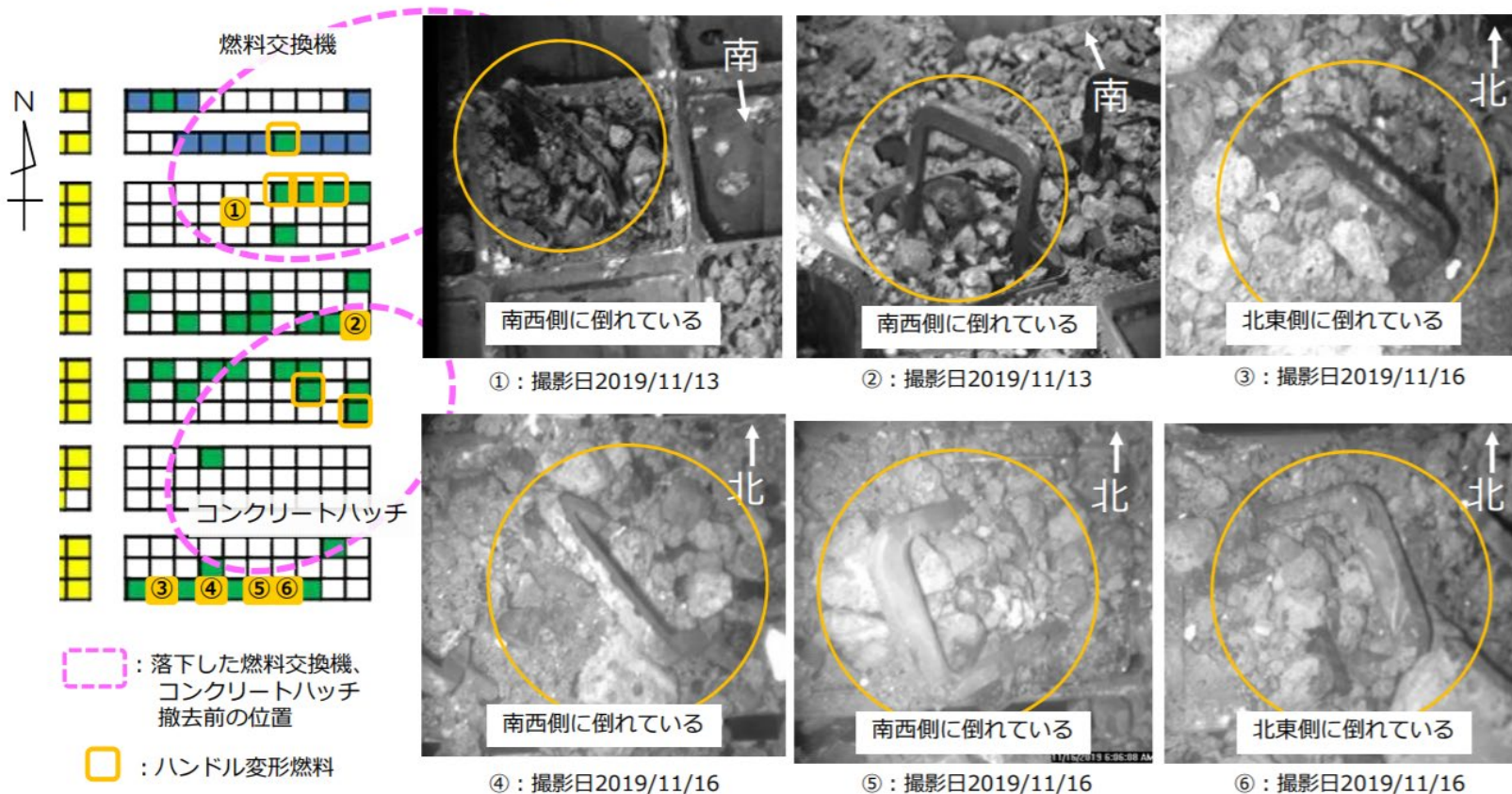
今回確認されたハンドル変形燃料
