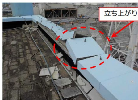
立ち上がり部材 (笠木) 状況
