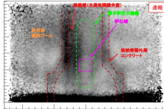
ミュオン測定による物質分布(密度長)の評価
