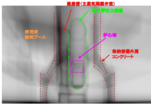
シミュレーションによる物質分布(密度長)の評価 (炉心域, および炉底部に燃料デブリありのケース)
